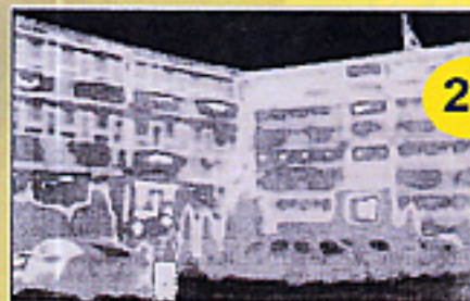
Wärmebild der Berufsschule mit erkennbaren Schwachstellen.
